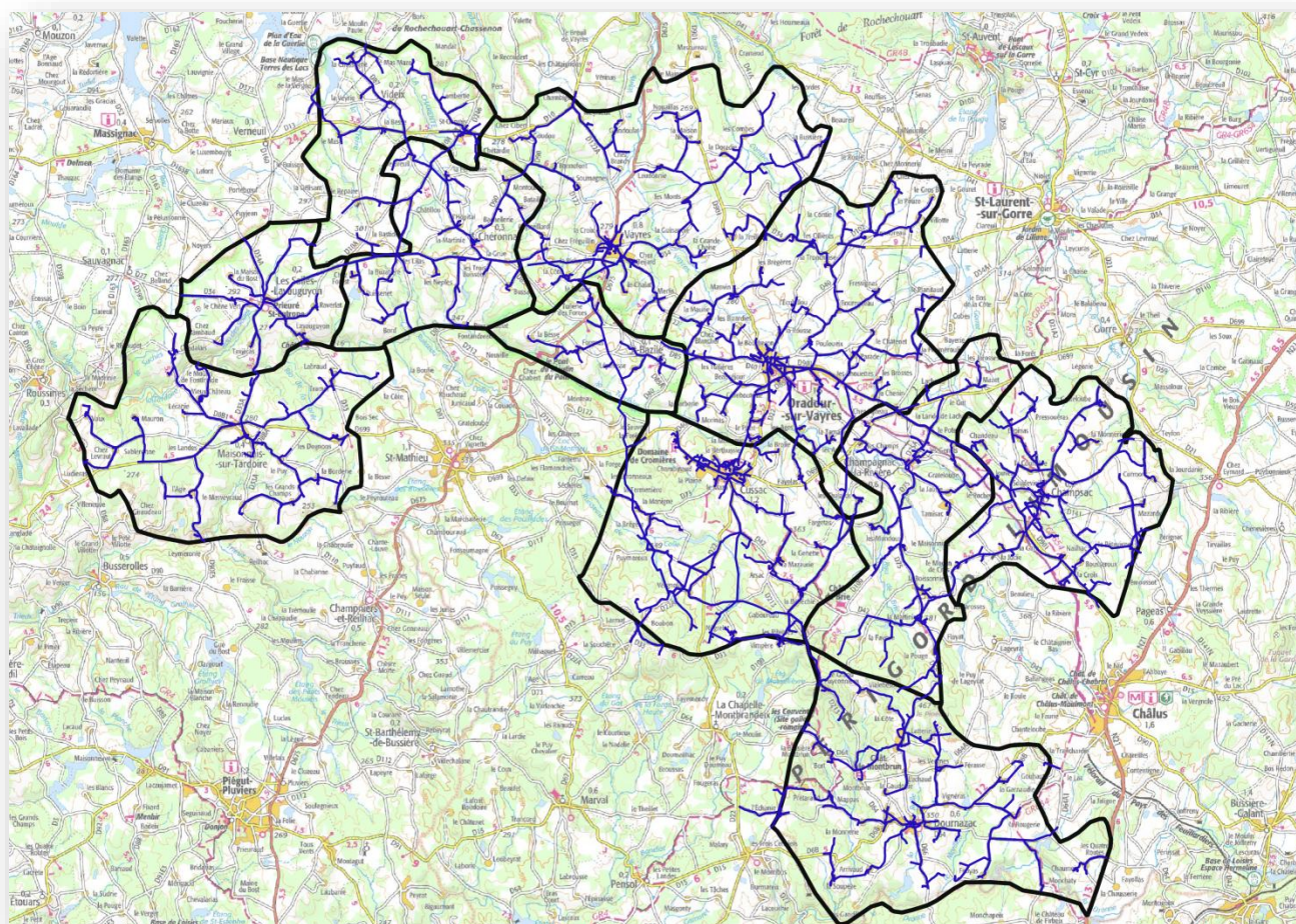
Figure 1 : réseau d'eau potable
